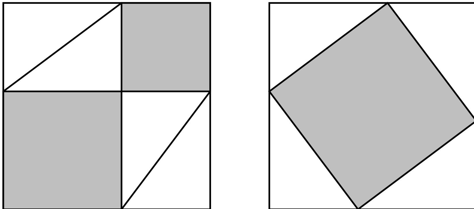
Figura 4.1: Dimostrazione del teorema di Pitagora.
