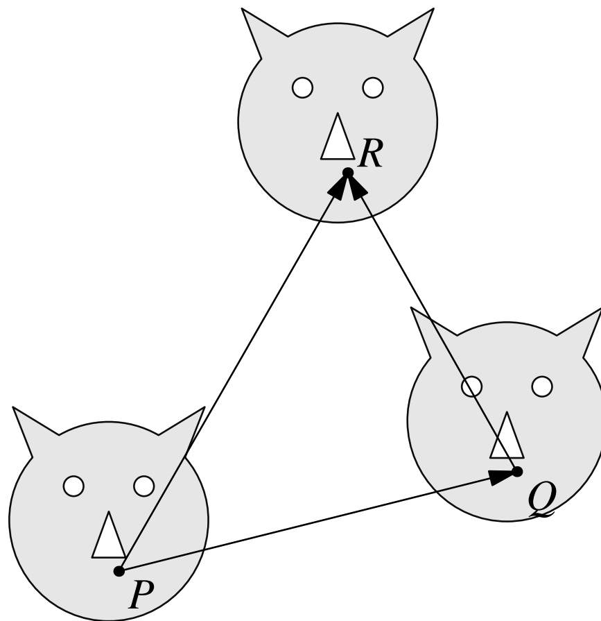
Figura 13.2: proprietà fondamentale degli spostamenti.
