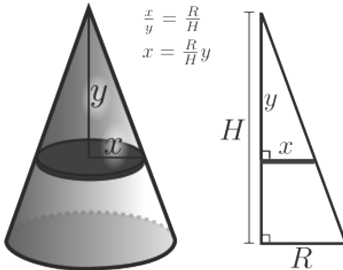
Figura 1.1: Volume del cono = \frac{1}{3}\pi R^2 H
