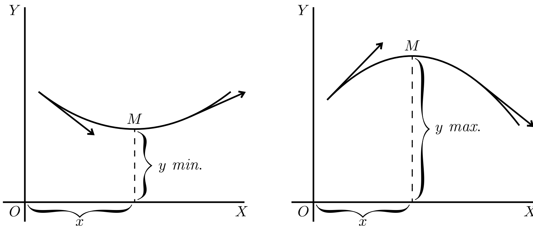
Figura 8.9: Massimi e minimi di una curva.
