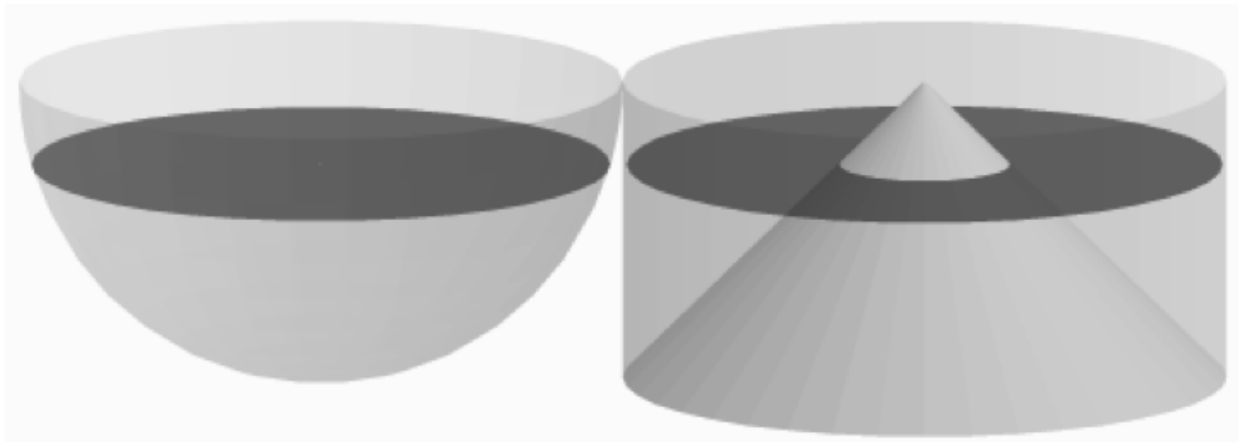
Figura 8.16: Costruzione per determinare il volume della sfera.
