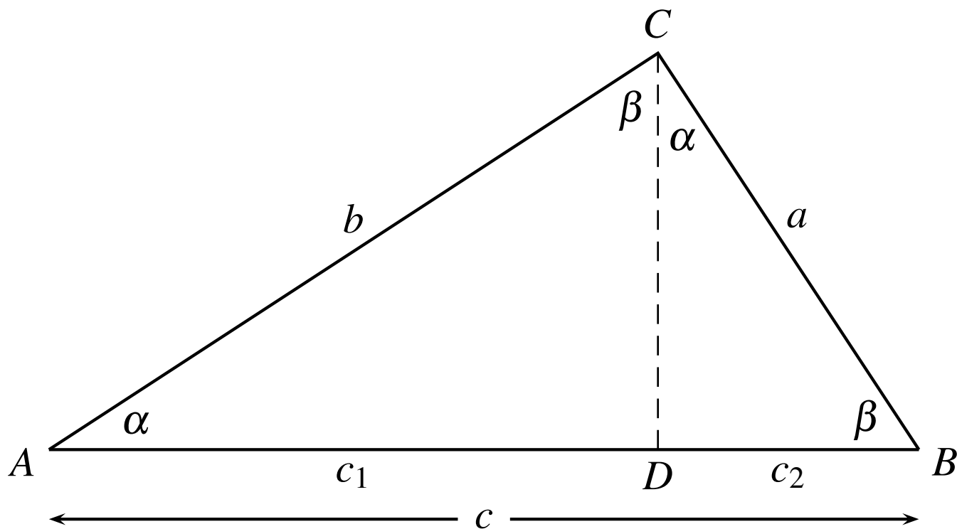
Figura 4.2: Dimostrazione “immediata” del teorema di Pitagora.
