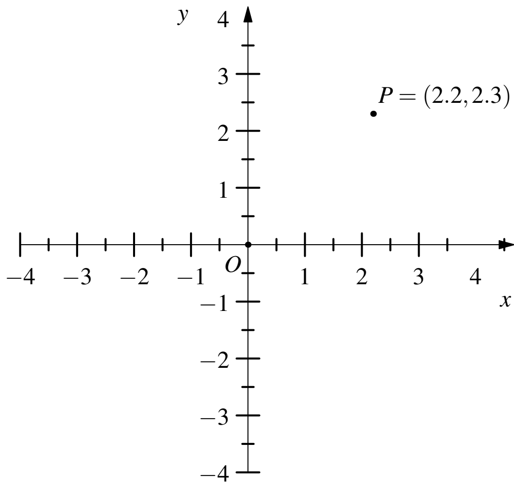
Figura 7.4: Coordinate cartesiane del piano.
