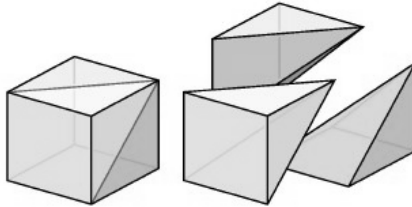
Figura 8.15: Il volume della piramide
