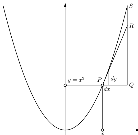
Figura 8.6: Calcolo della derivata.
