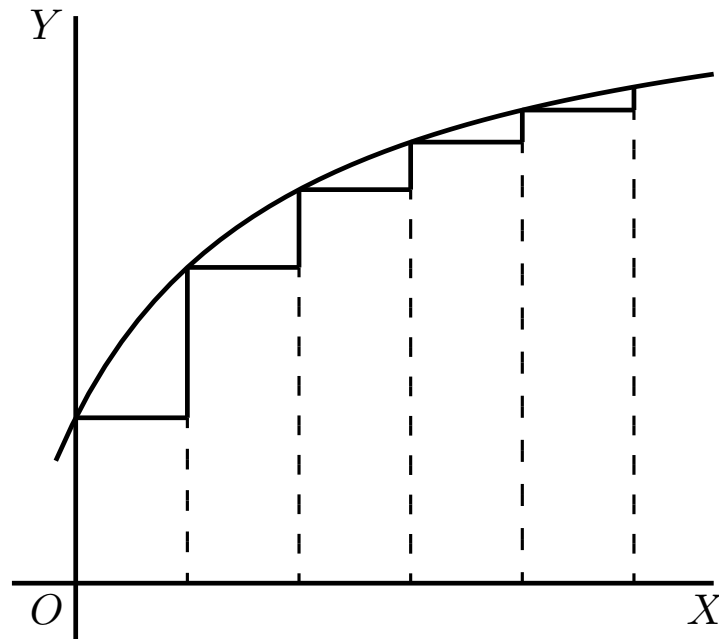
Figura 8.8: Derivata seconda negativa: la pendenza diminuisce.
