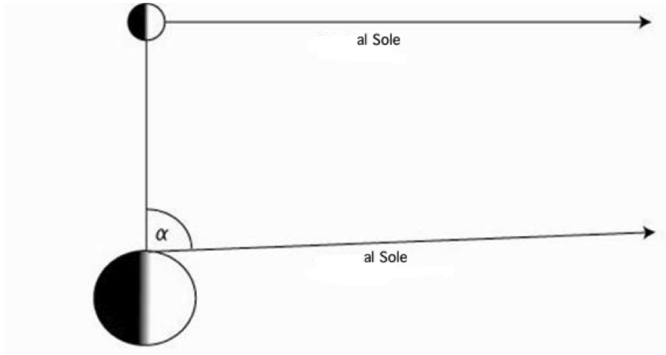
Figura 5.3: Geometria per il calcolo della distanza Terra-Sole.
