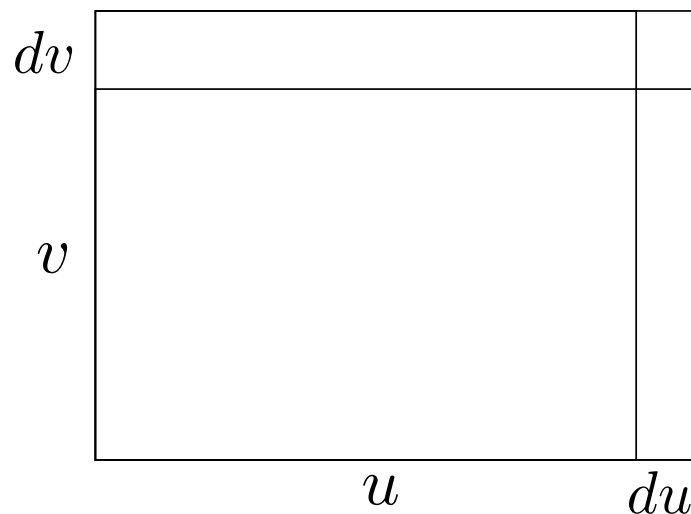
Figura 8.5: Illustrazione della regola (4).
