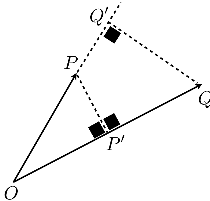
Figura 13.5: Il prodotto scalare del vettore \mathbf{a} = \vec{OP} con il vettore \mathbf{b} = \vec{OQ} è uguale a |OP| \cdot |OQ'| , dove OQ' è la proiezione ortogonale di \vec{OQ} su \vec{OP} . (il simbolo ■ denota un angolo retto). Con un semplice ragionamento geometrico si verifica che |OP| \times |OQ'| = |OQ| \cdot |OP'| e quindi che il prodotto scalare è simmetrico, \mathbf{a} \bullet \mathbf{b} = \mathbf{b} \bullet \mathbf{a} .
