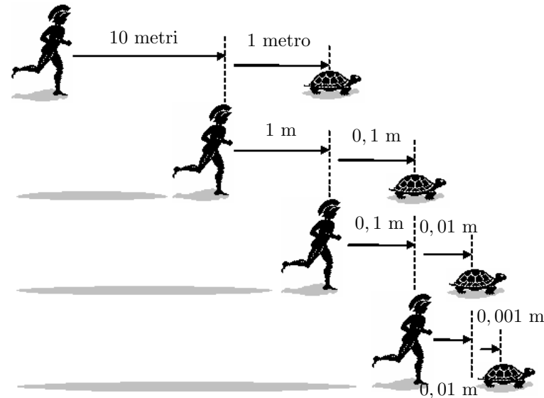
Figura 10.1: Achille e la tartaruga.
