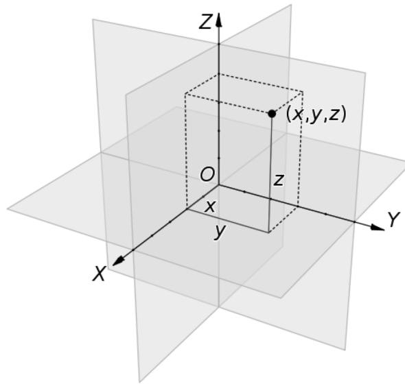
Figura 13.4: Coordinatizzazione dello spazio.
