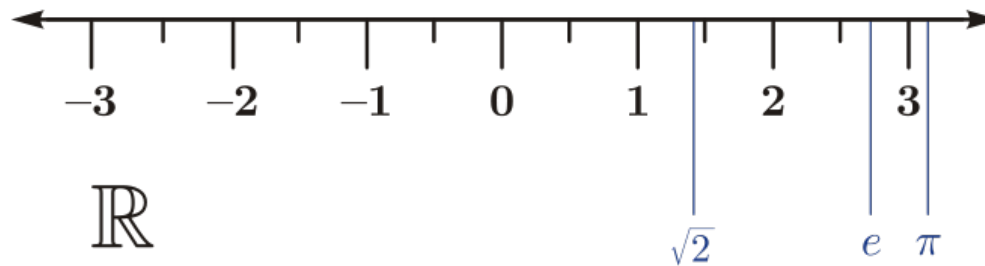
Figura 7.2: la retta numerica o retta reale.
