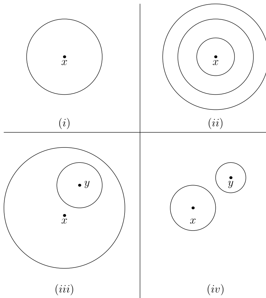
Figura 17.2: Illustrazione dei 4 assiomi di Hausdorff.
