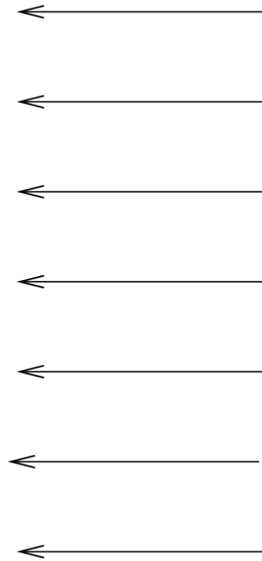
Figura 5.1: La figura mostra il procedimento seguito da Eratostene per calcolare la dimensione del raggio della Terra.
