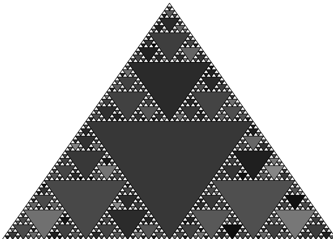
Figura 9.3: Triangolo di Sierpinski.
