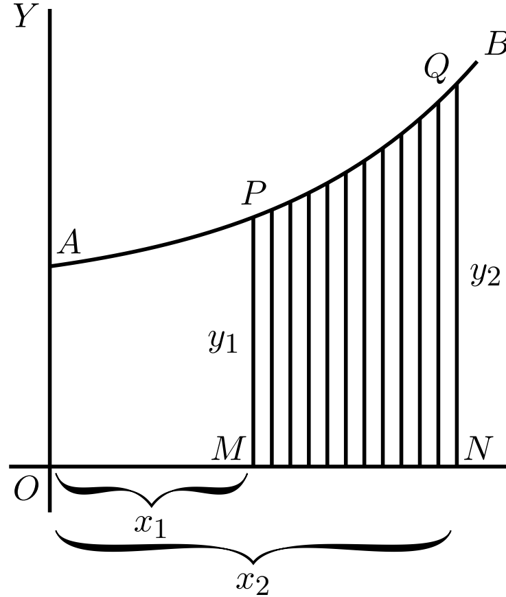
Figura 8.10: Significato geometrico dell'integrale
