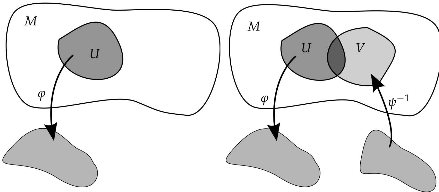
Figura 17.4: Nozione moderna di molteplicità M o varietà.
