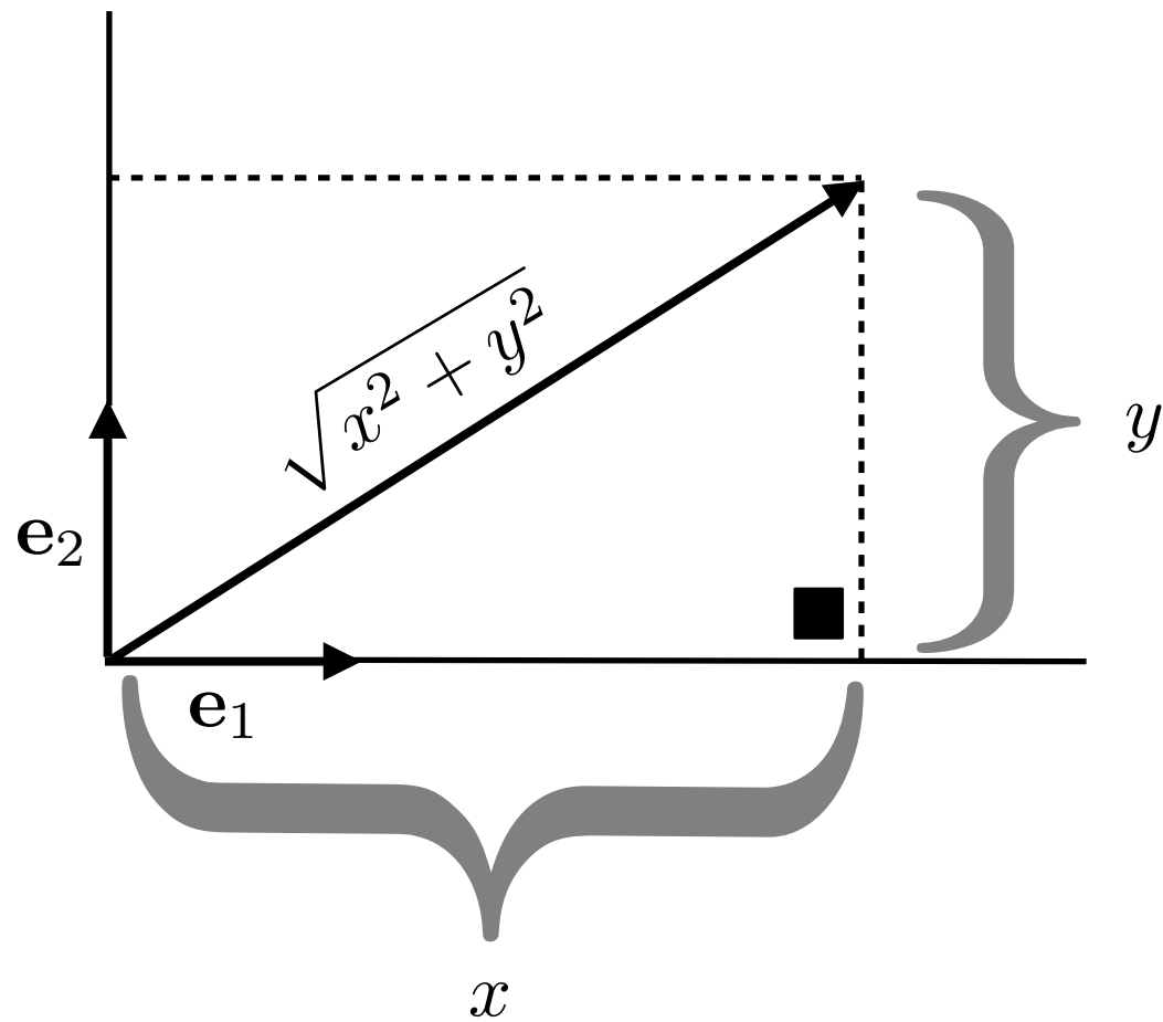
Figura 13.6: Coordinate cartesiane e teorema di Pitagora.
