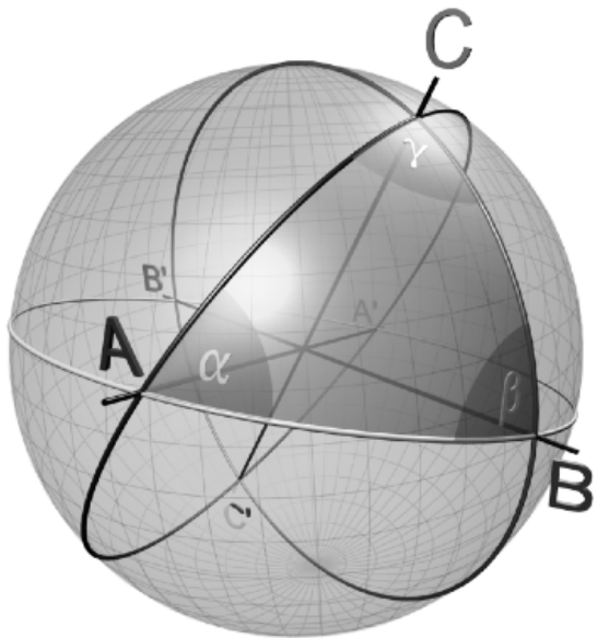
Figura 16.2: Triangoli geodetici su una 2-sfera e su una superficie con curvatura costante negativa.
