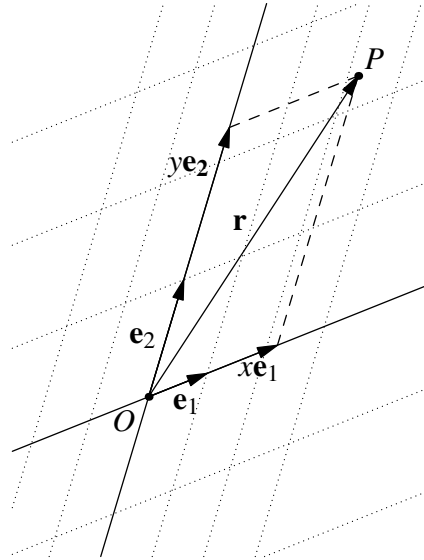
Figura 13.3: Coordinatizzazione del piano.
