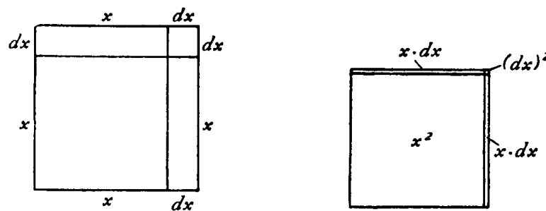
Figura 8.4: Significato geometrico della regola fondamentale del calcolo.
