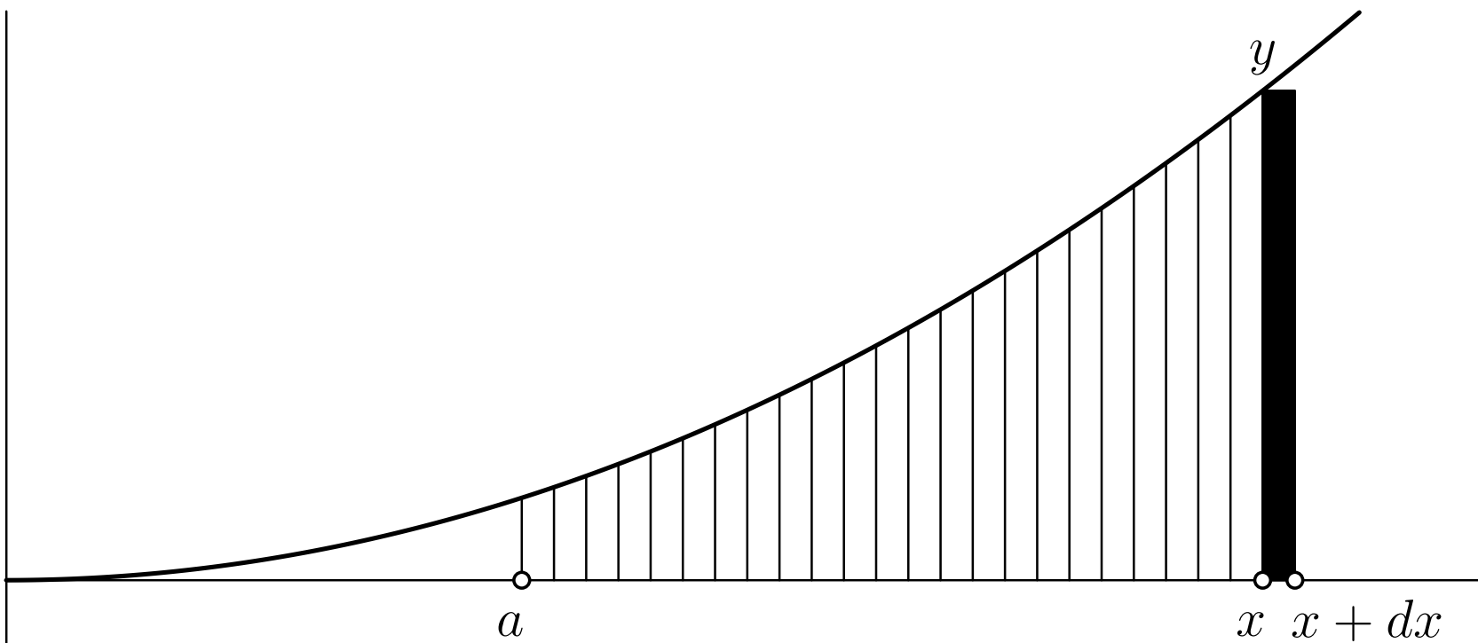
Figura 8.12: Calcolo della derivata.
