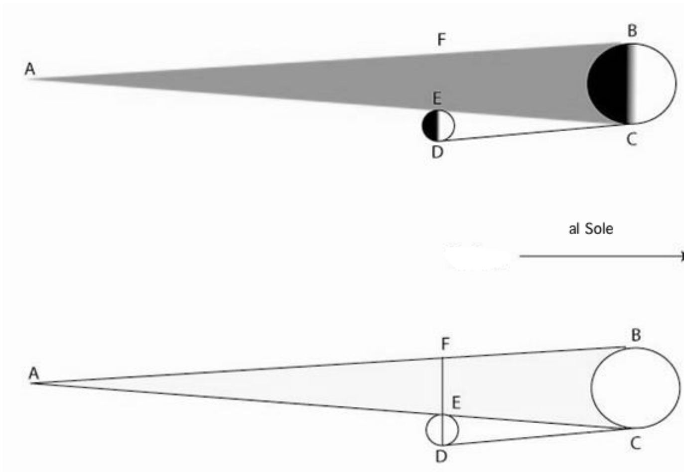
Figura 5.2: Geometria dell'eclisse lunare.
