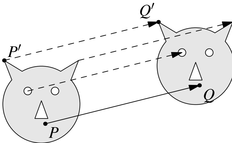
Figura 13.1: Spostamento rigido di una figura nel piano.
