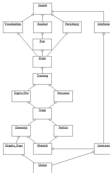
Fig. 1. Geant4 kernel
