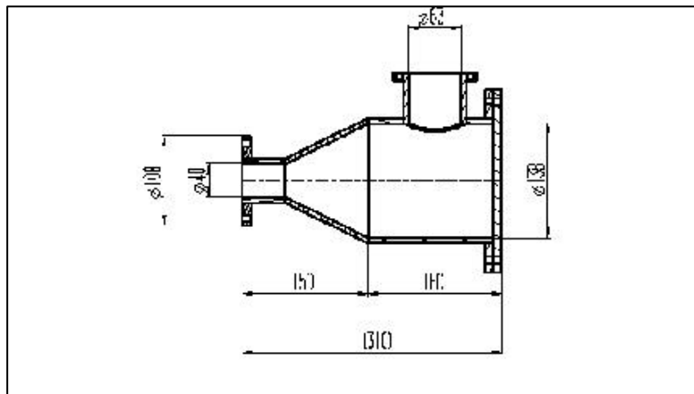
Fig. 6 : intermediate JB cross section (proposal).
